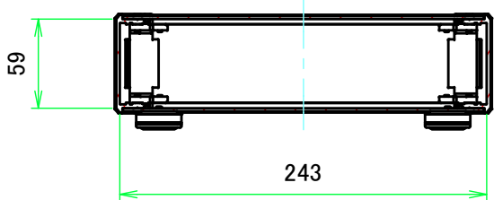
B-B ( 1:4.5 )
